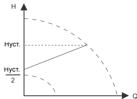
Рис. 18 Пропорциональное давление
