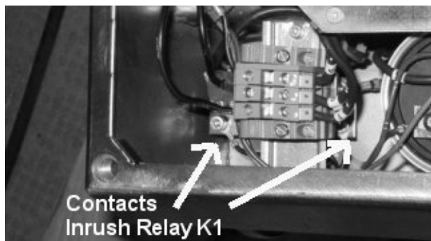
Рис. 9 Реле K1 ограничения пускового броска тока
