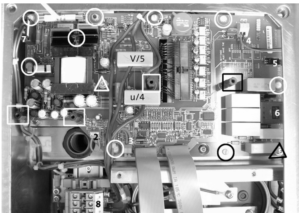
Рис. 32 Винты платы блока питания
