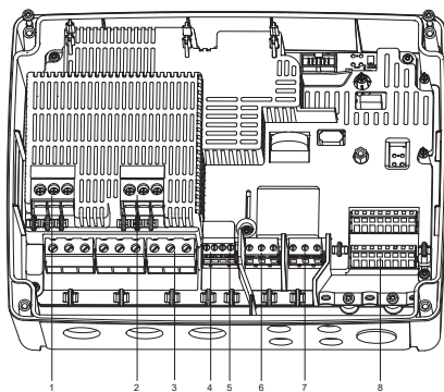
4-сүр. Клеммалар
