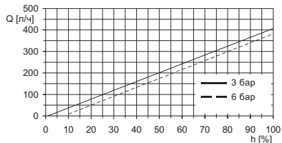
Рис. 66 DMX 321-6 (60 Гц)
