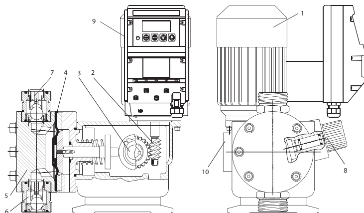
Рис. 1 DMX 226
