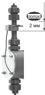
Рис. 16 Контроллер дозирования
