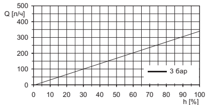
Рис. 67 DMX 321-4 (50 Гц)
