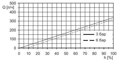
Рис. 65 DMX 321-6 (50 Гц)
