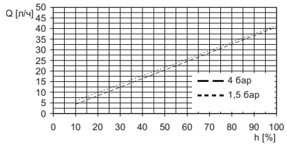
Рис. 37 DMX 37-5 (50 Гц)
