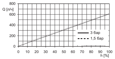
Рис. 75 DMX 525-3 (50 Гц)
