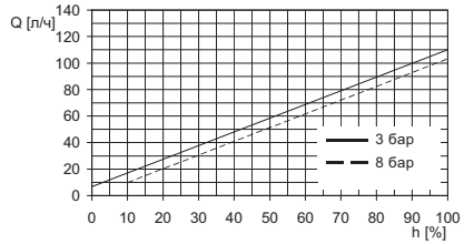
Рис. 34 DMX 100-8 (50 Гц)
