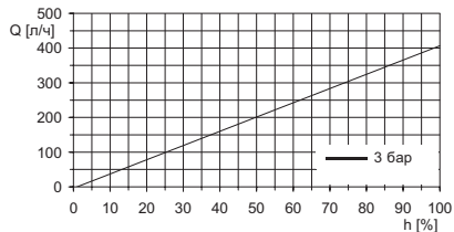
Рис. 68 DMX 321-4 (60 Гц)
