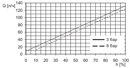
Рис. 35 DMX 100-8 (60 Гц)
