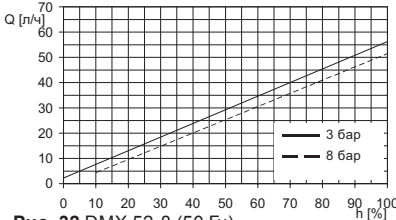
Рис. 32 DMX 52-8 (50 Гц)
