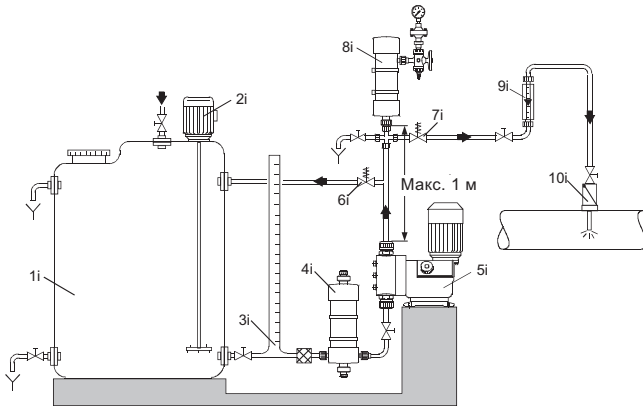
4-сур. Оңтайлы монтаж мысалы
