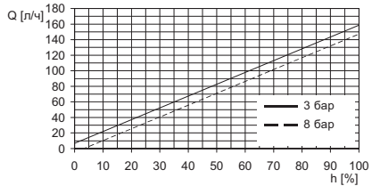
Рис. 36 DMX 142-8 (50 Гц)
