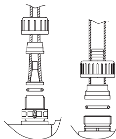
Рис. 13 Подключение шлангов
