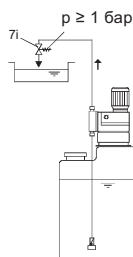
11-сур. Қысымды сақтау клапанымен орнату
